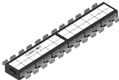
Адаптерная сборка EHD MPO Adapter Pack
